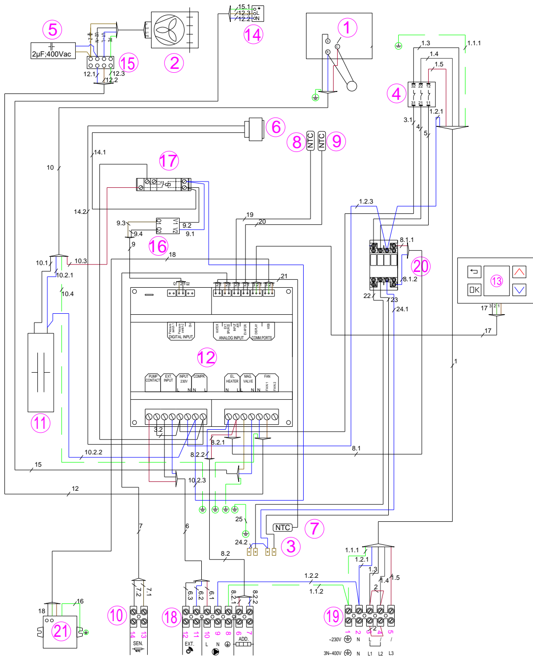
Abbildung 15: Elektrischer Schaltplan
