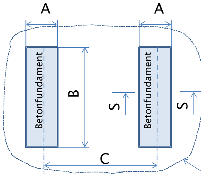
Draufsicht
