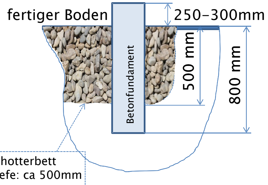
Schnitt S-S
